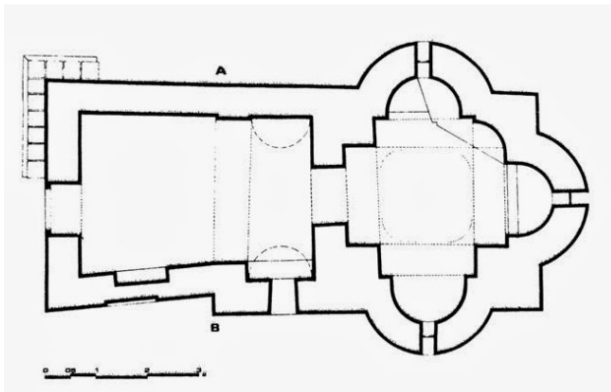
Σχεδιαστική κάτοψη της Παναγίας Κουμπελίδικης.
