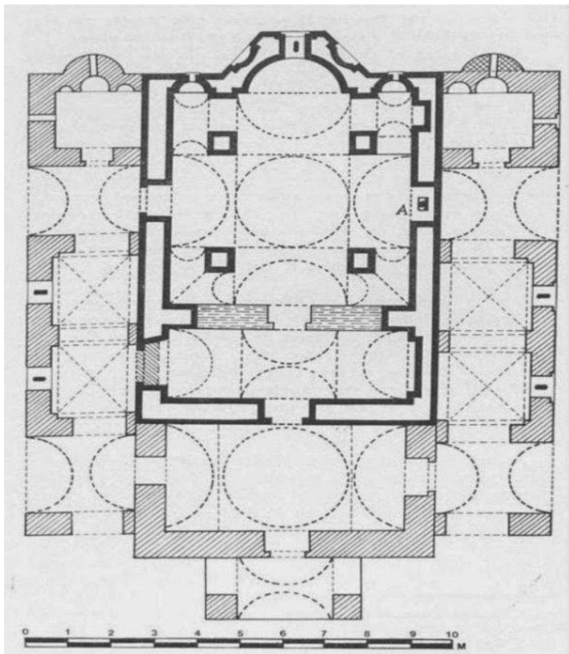
Κάτοψη του βυζαντινού ναού του Αγίου Γεωργίου στην Ομορφοκκλησιά Καστοριάς. Με το Α η θέση της γλυπτής εικόνας του Αγίου Γεωργίου.
